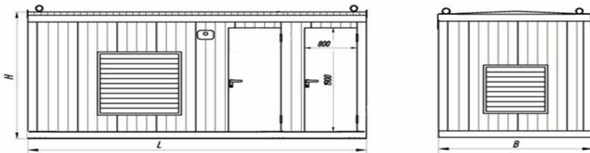
Рисунок 2. Общий вид стандартных контейнеров ПБК 3 - 8
